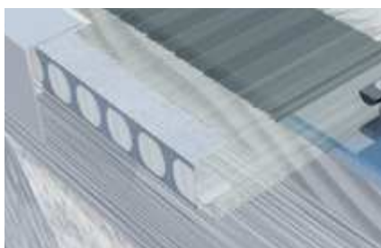
3 AntiDUST® tape und U-Profil Zur Abdichtung der offenen Paneeelseiten. Die Variante mit Filter gehört an das untere Plattenende, damit das Kondenswasser ablaufen kann.
