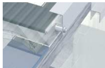
4 Reinaluminium-Klebeband Die der Platte zugewandten Oberflächen müssen reflektierend oder hell sein. Alternativ zum Alu-Klebeband ist auch ein Anstrich mit weißer Dispersions- oder Acrylfarbe auf Wasserbasis möglich. Der Anstrich muss gut ausgetrocknet sein.
